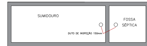
PLANTA BAIXA-FOSSA E SUMIDOURO
