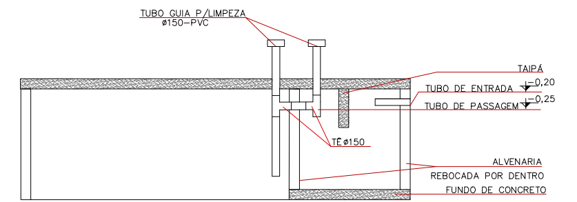
CORTE-FOSSA E SUMIDOURO
