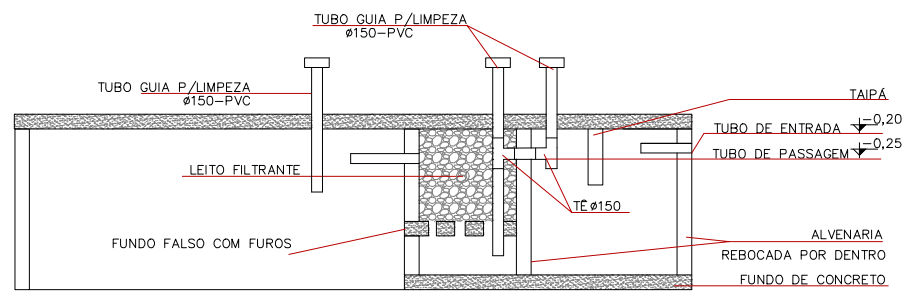
CORTE-FOSSA, FILTRO E SUMIDOURO
