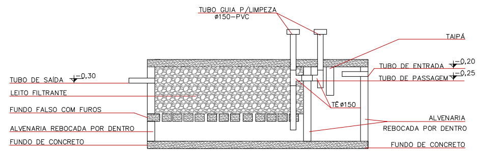
CORTE-FILTRO E FOSSA
