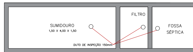
PLANTA BAIXA-FOSSA, FILTRO E SUMIDOURO
