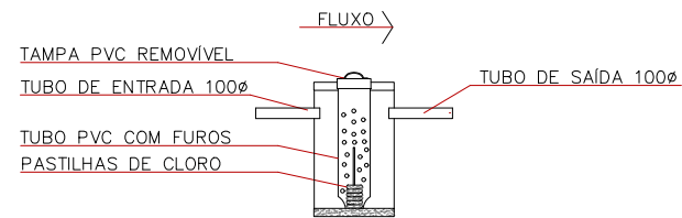
CORTE-CLORADOR
