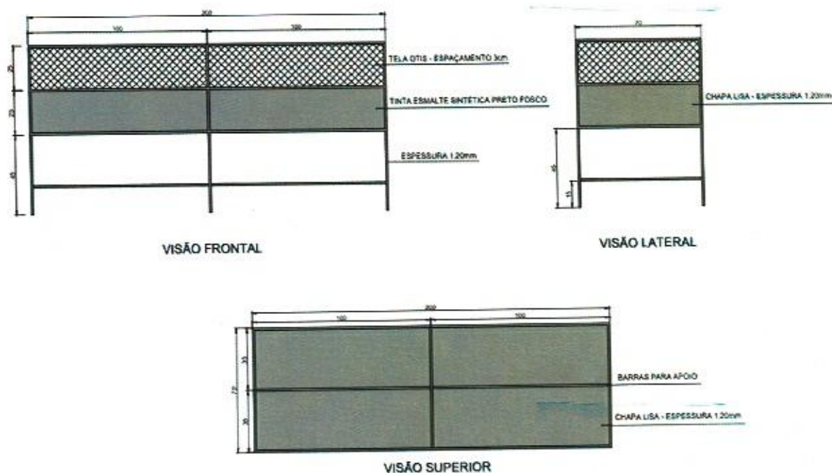
Imagem 1 – Projeto modelo das lixeiras públicas
