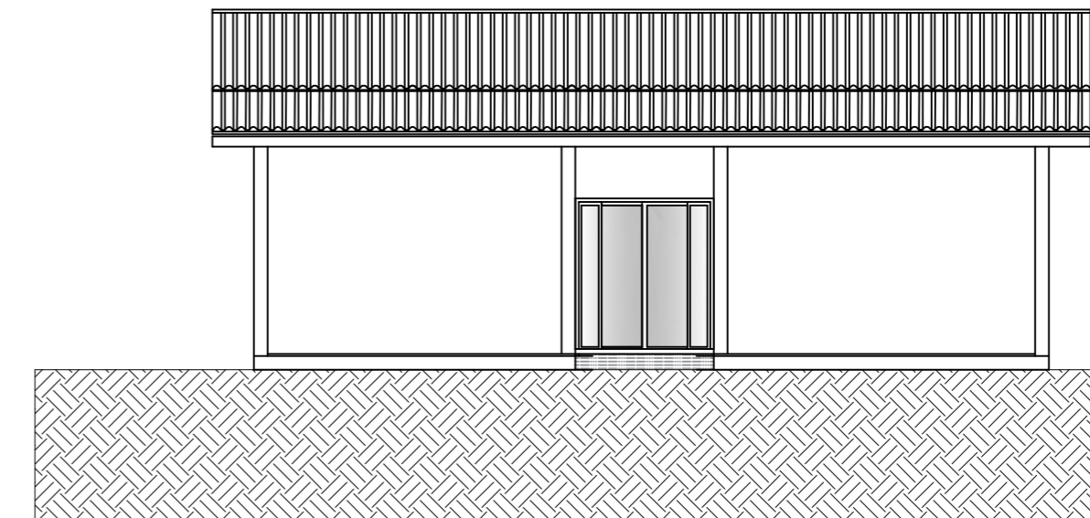
FACHADA SUL ESCALA 1:50
