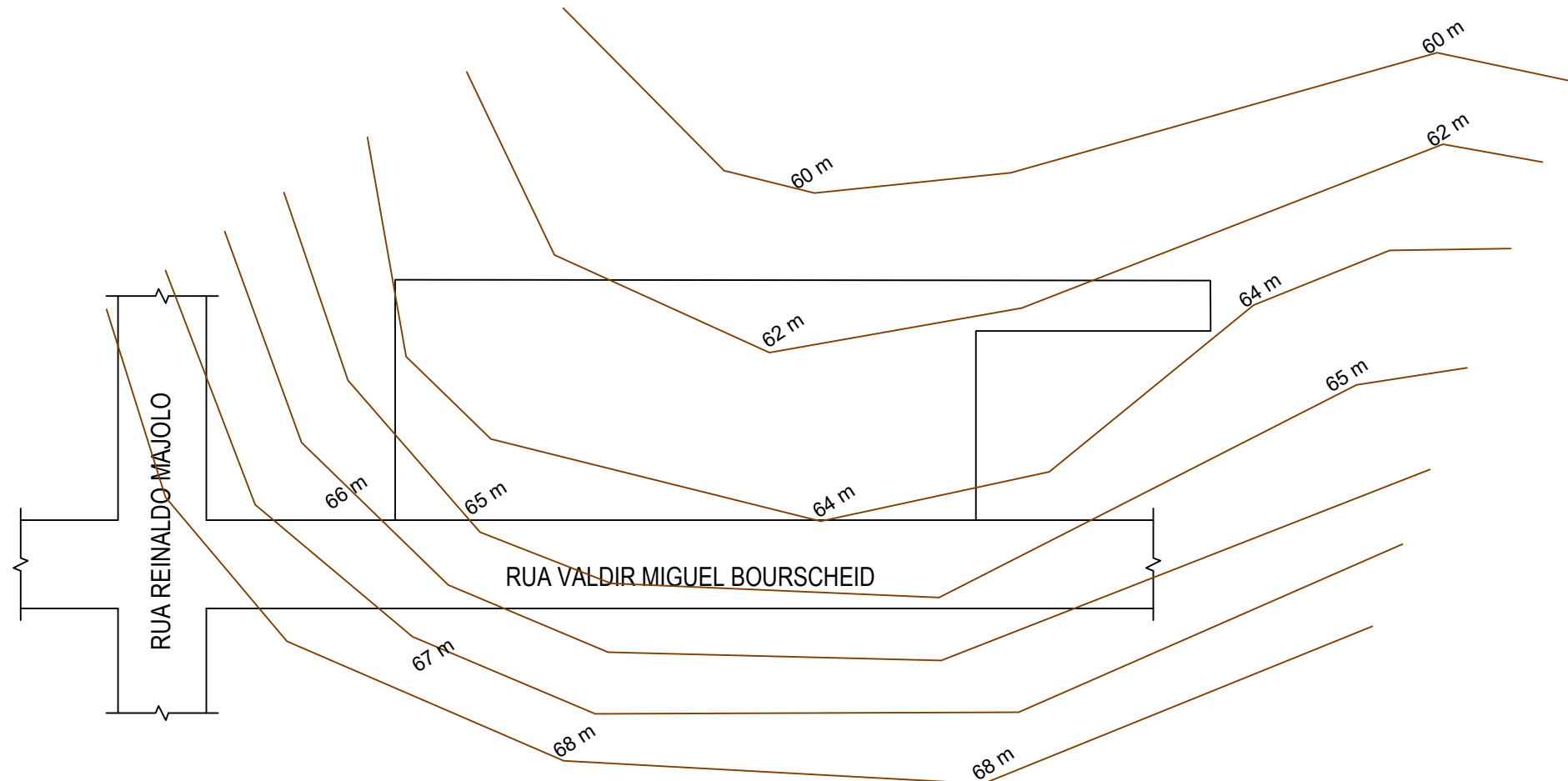
PLANTA DE LEVANTAMENTO PLANIALTIMÉTRICO ESCALA 1:1000
