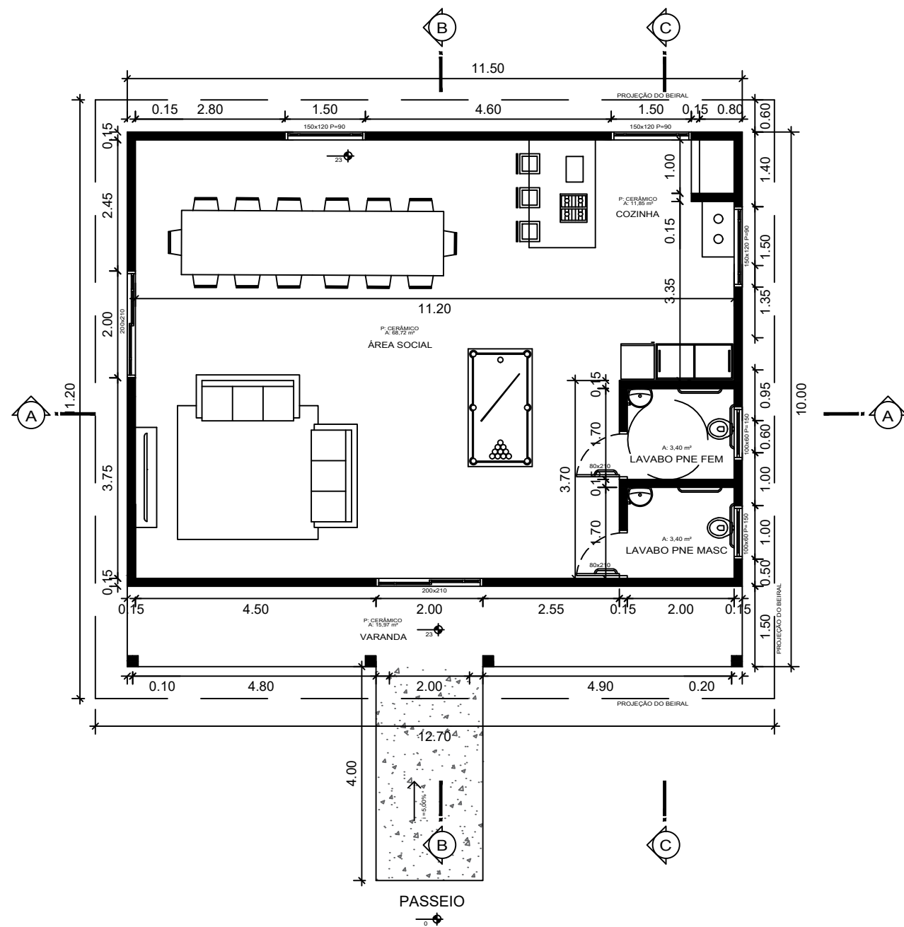
PLANTA BAIXA - ÁREA 115,00 m 2 ESCALA 1:50
