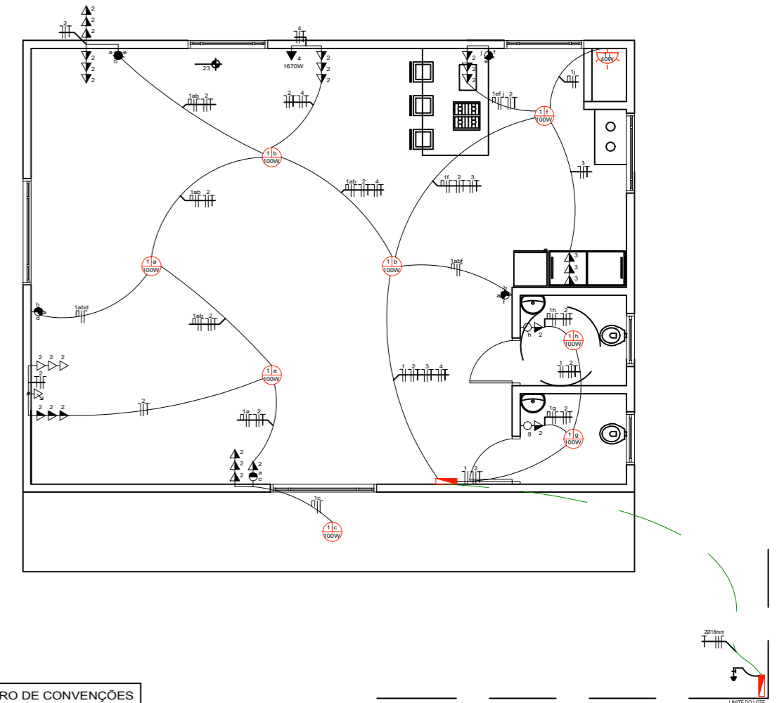
PROJETO ELÉTRICO ESCALA 1:50
