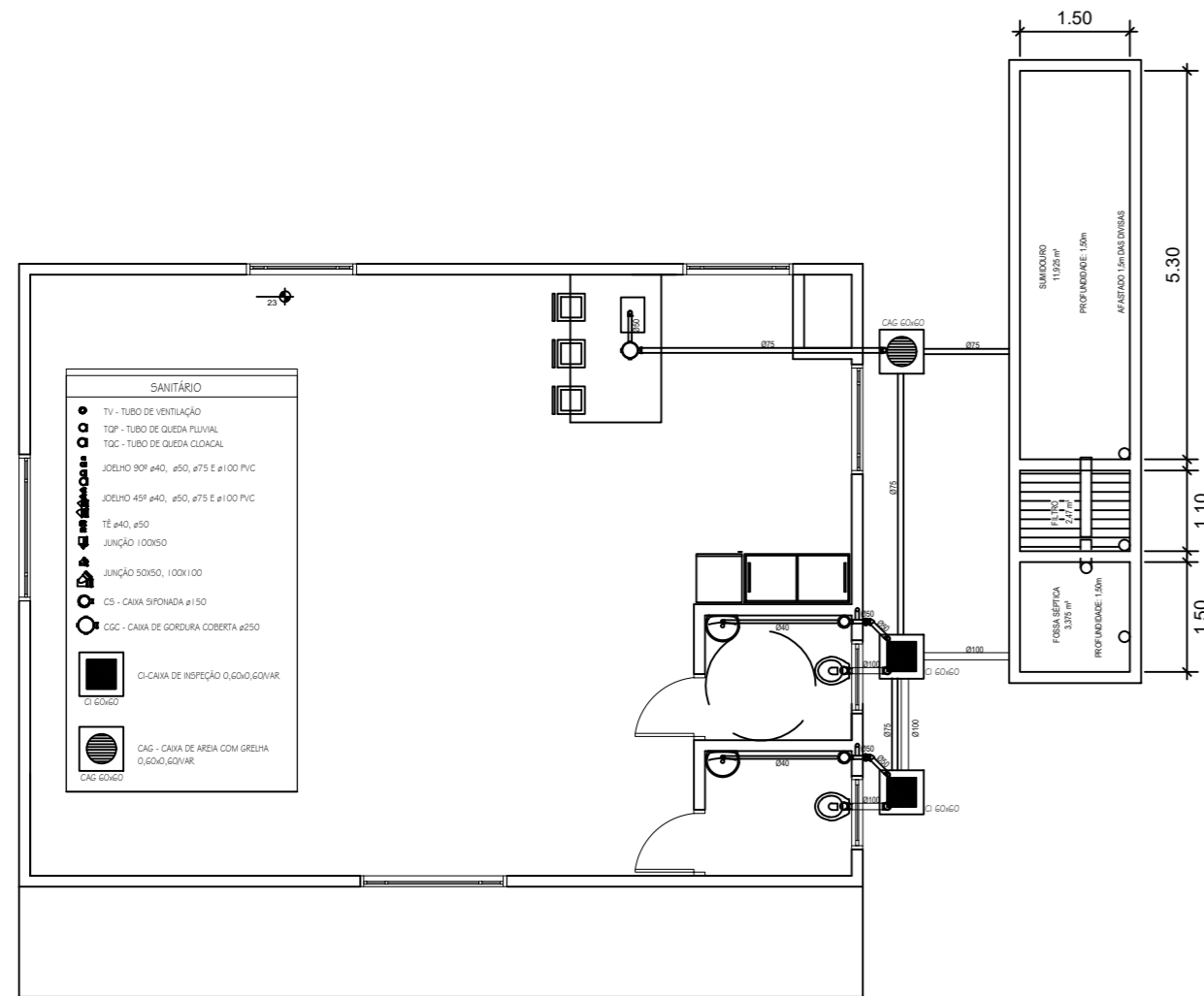
PROJETO SANITÁRIO ESCALA 1:50
